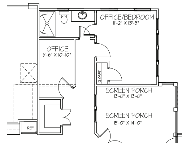
Optional office nook
